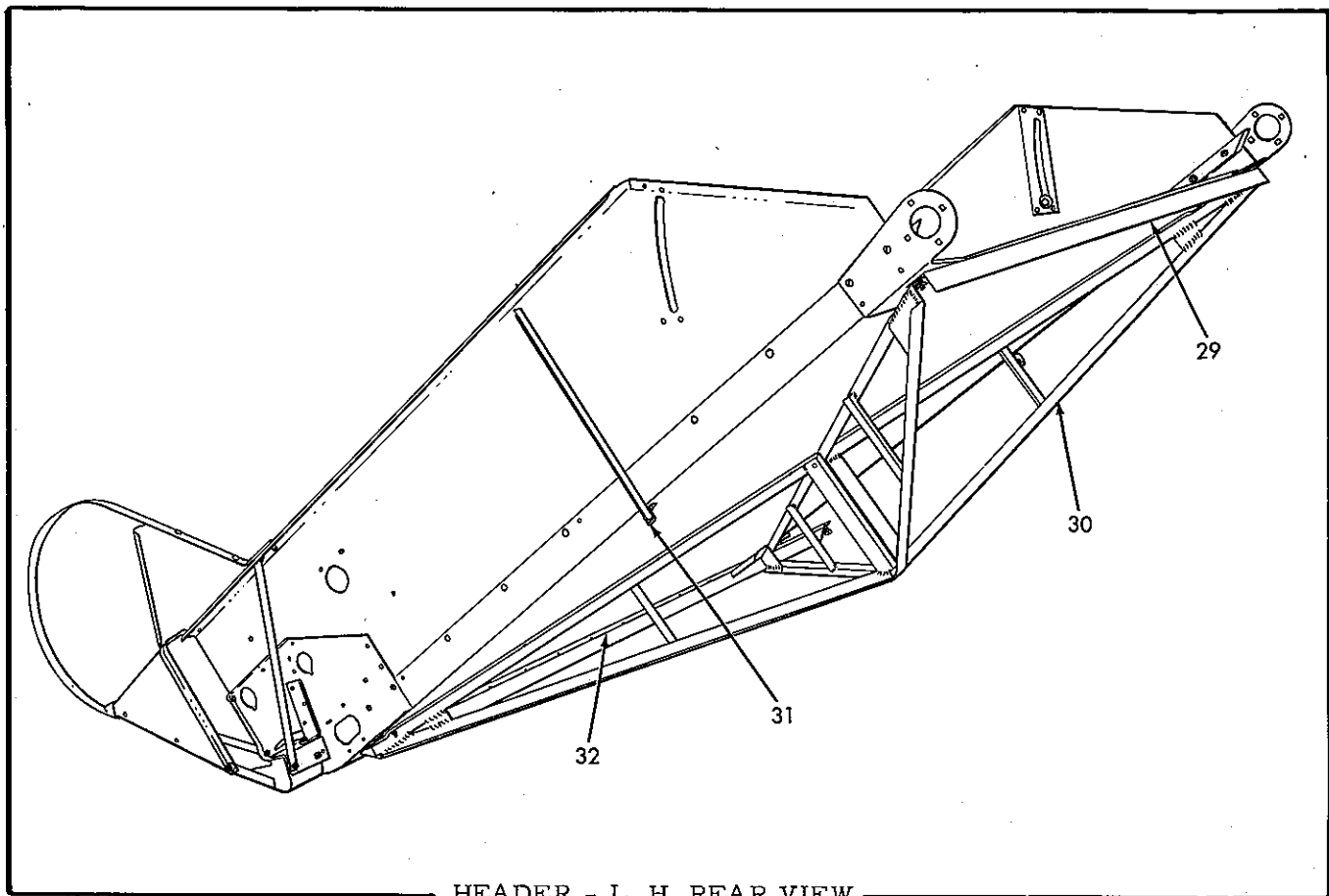
HEADER - L. H. REAR VIEW
